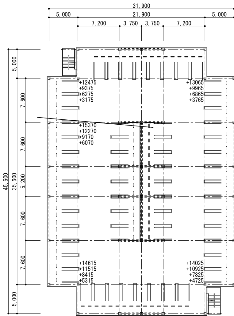
2~5階平面図
