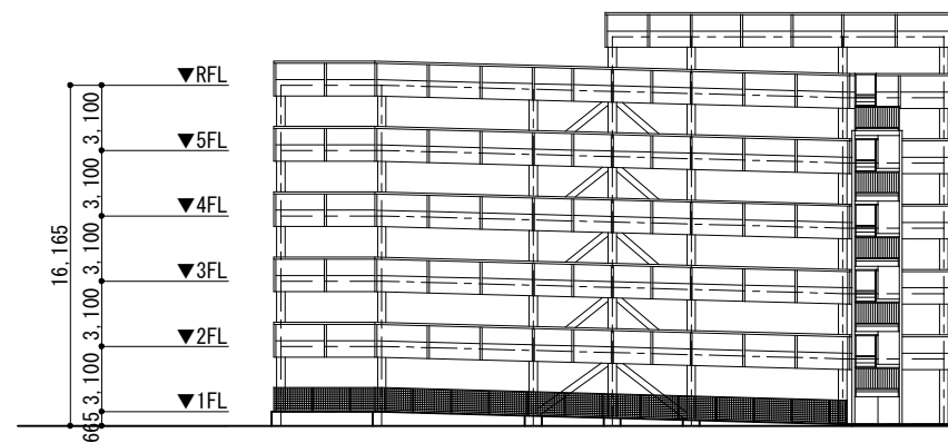
北側立面図
