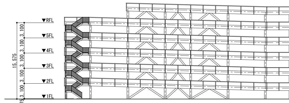
西側立面図
