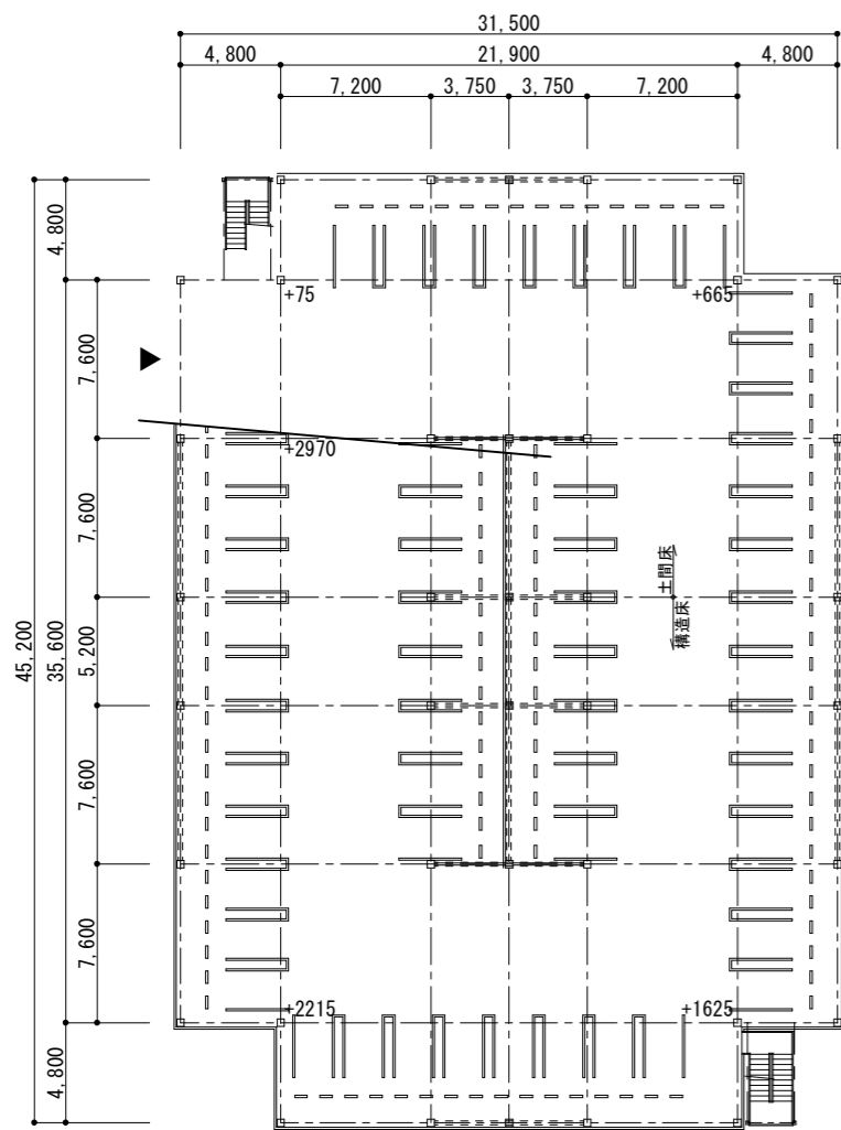
1階平面図
