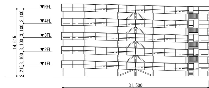
南側立面図
