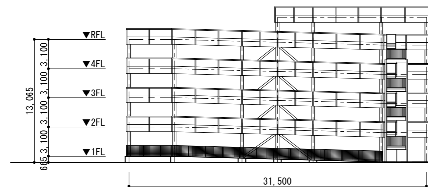
北側立面図
