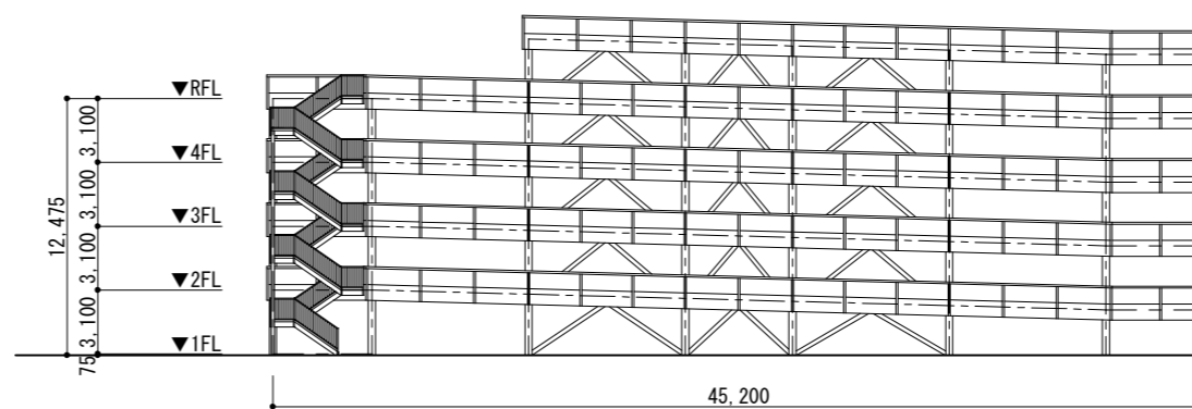
西側立面図
