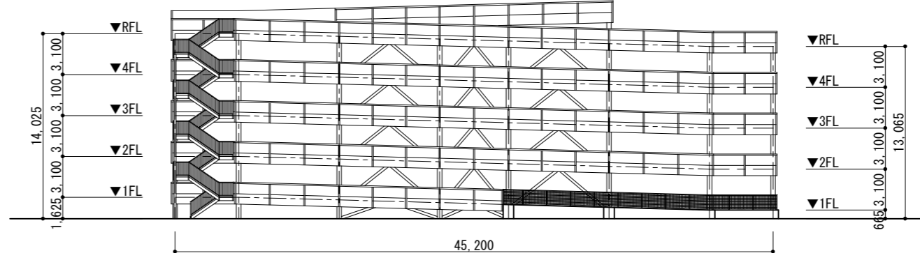
東側立面図
