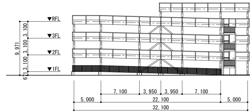
北側立面図
