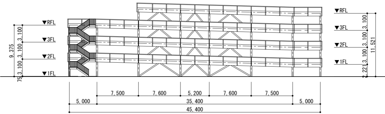
西側立面図
