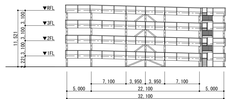
南側立面図
