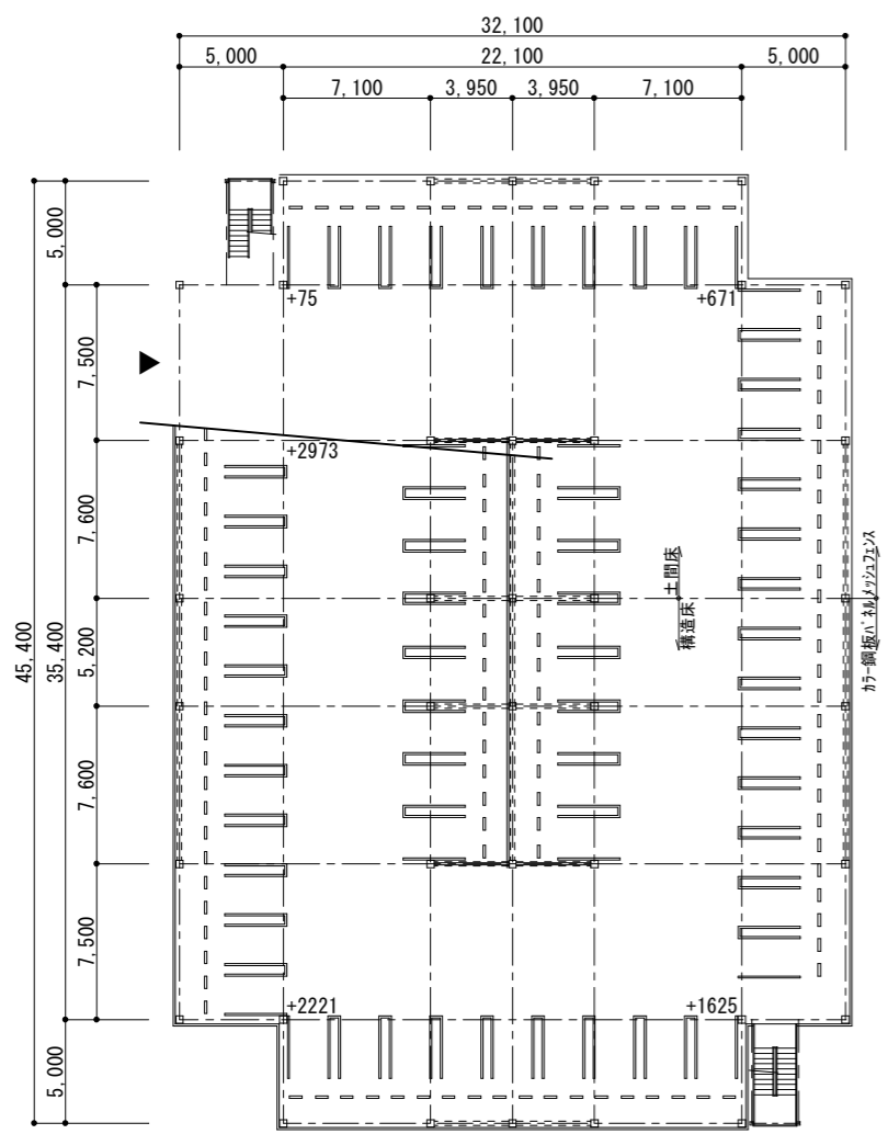
1階平面図
