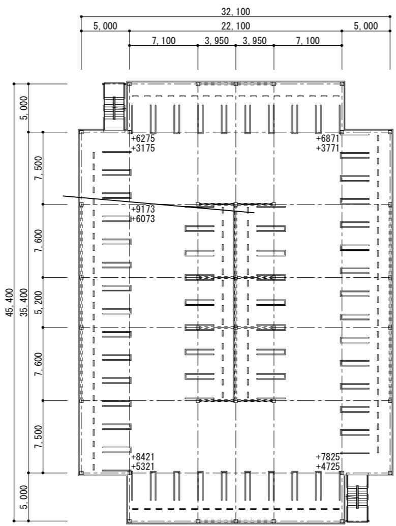
2・3階平面図
