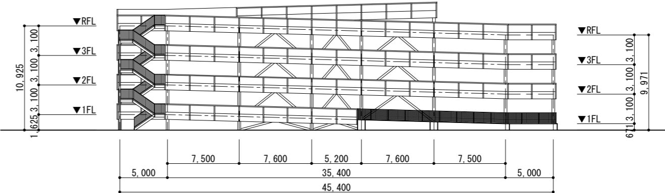
東側立面図
