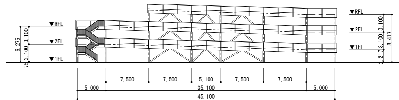
西側立面図
