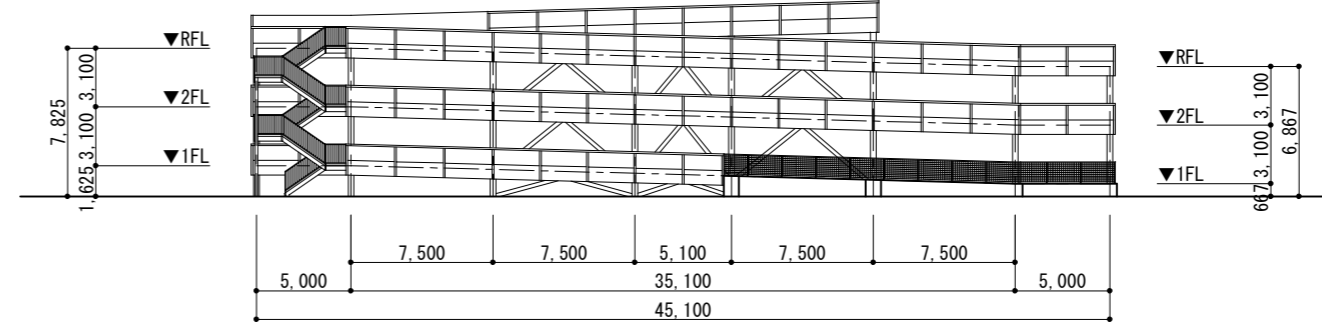
東側立面図
