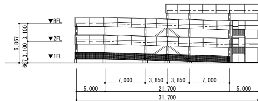
北側立面図
