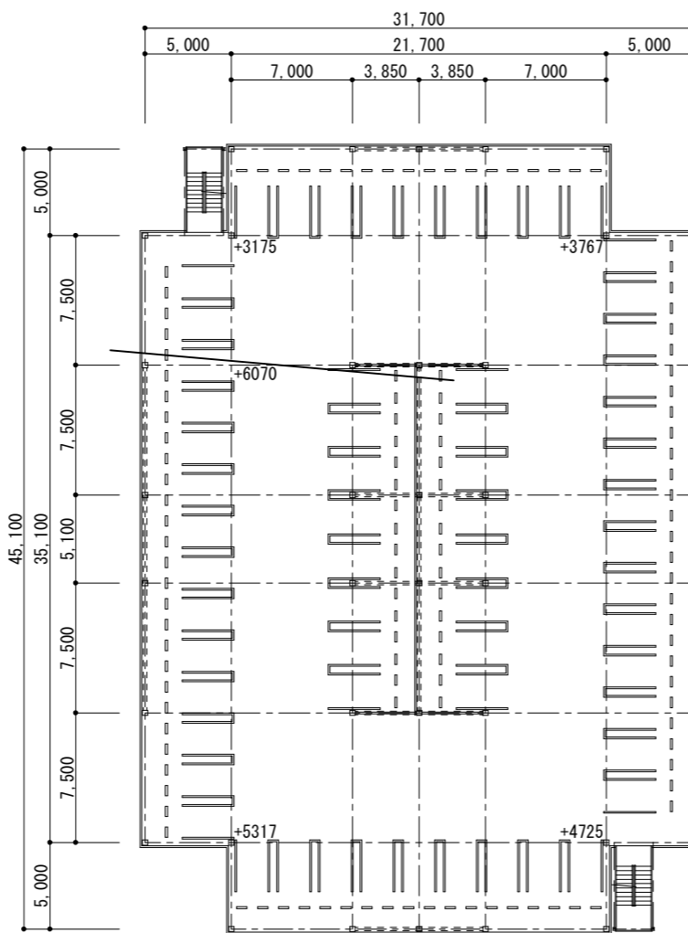
2階平面図
