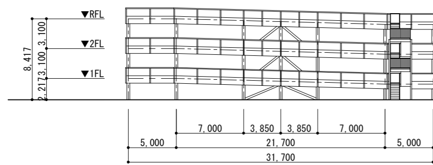
南側立面図
