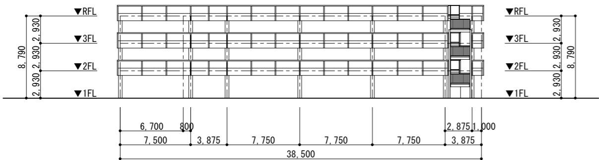
南側立面図
