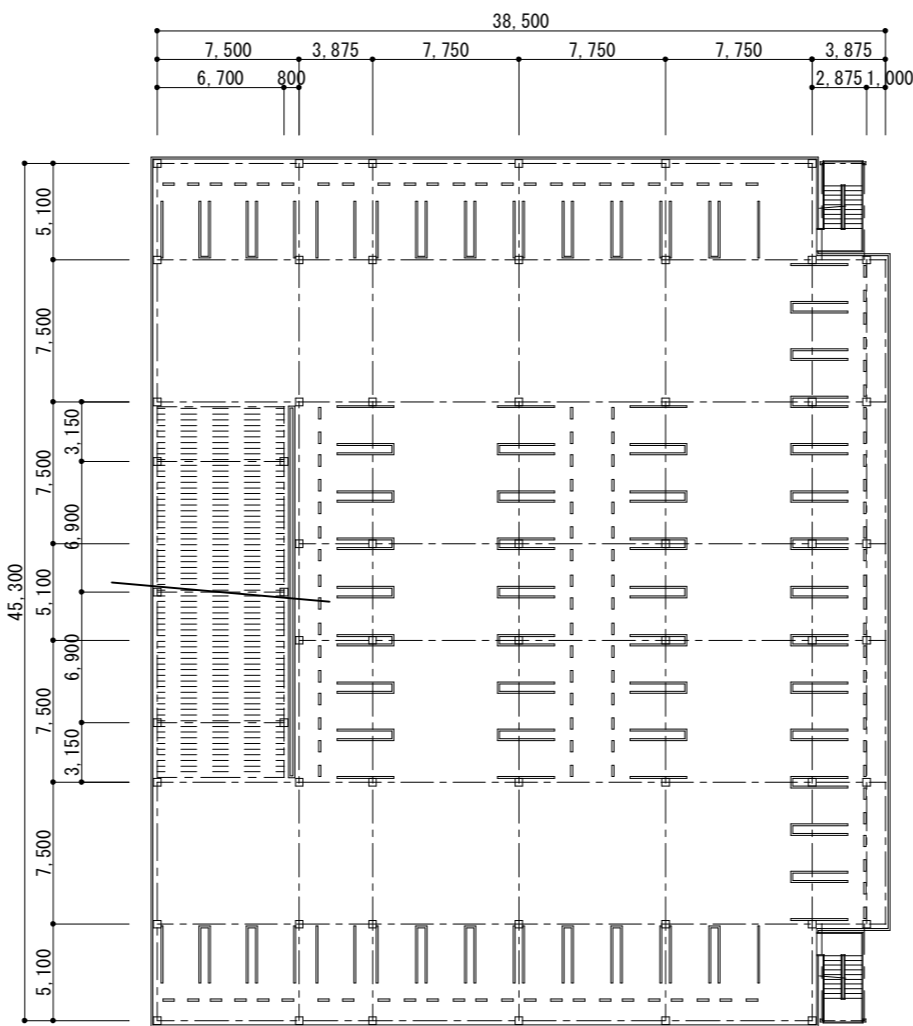
2・3階平面図
