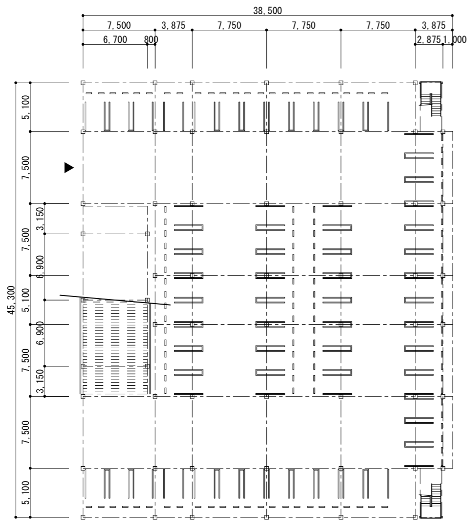
1階平面図
