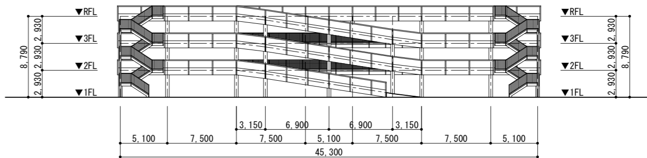
西側立面図
