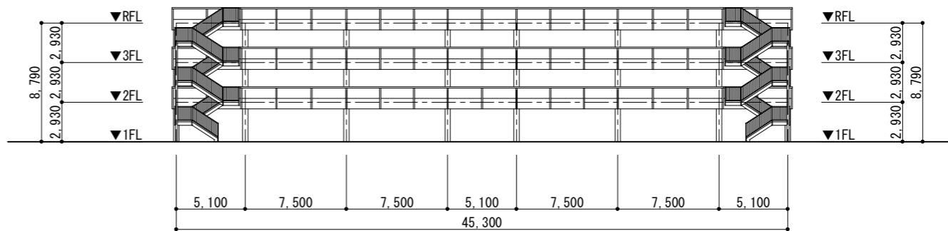
東側立面図
