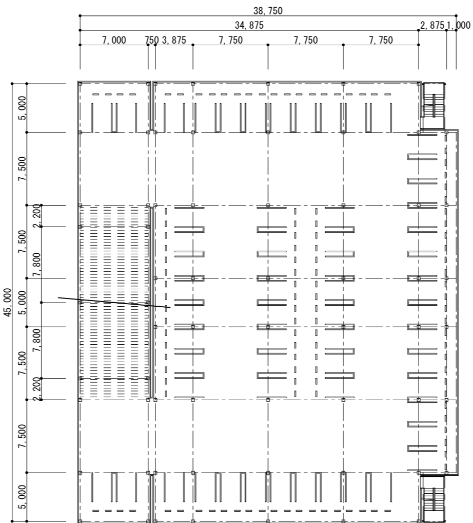
2階平面図
