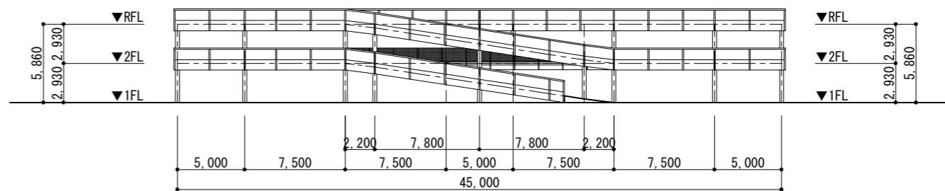
西側立面図
