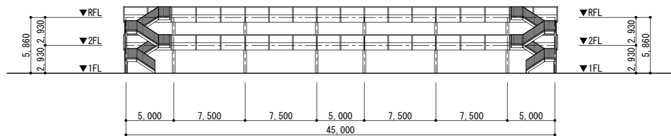
東側立面図
