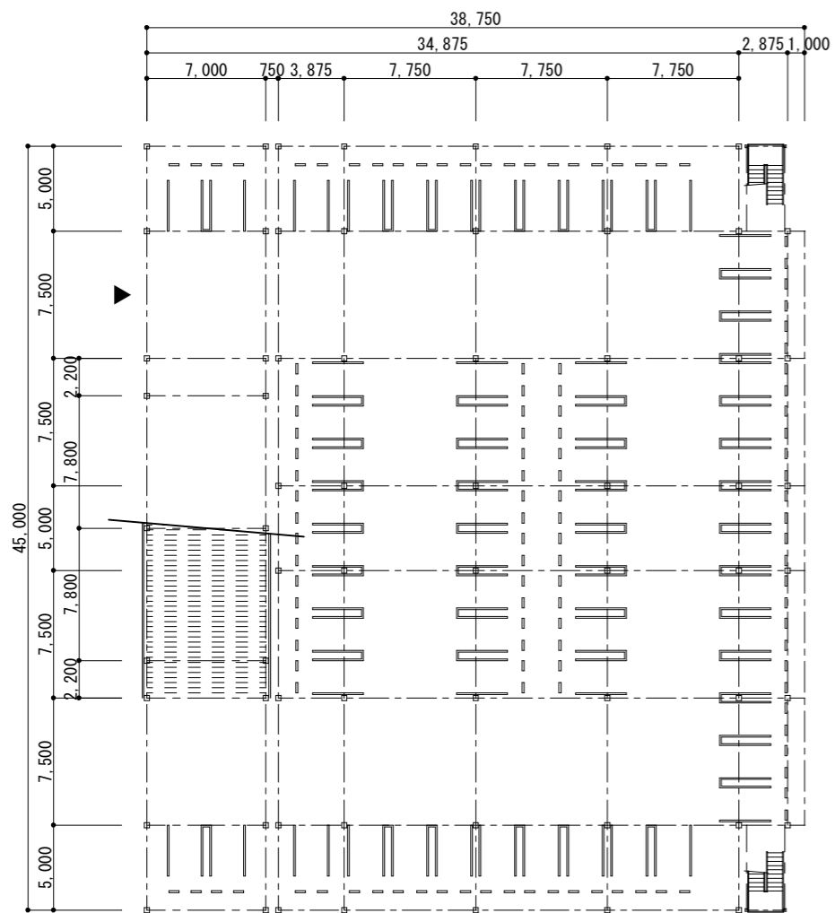
1階平面図
