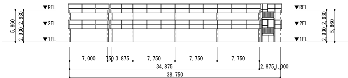
南側立面図
