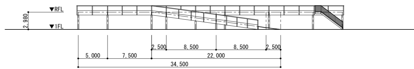
西側立面図
