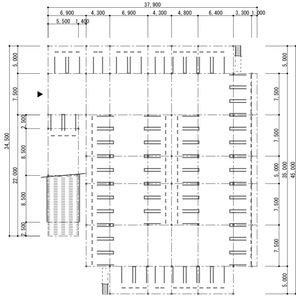
1階平面図
