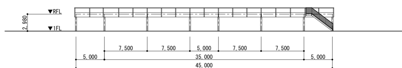
東側立面図
