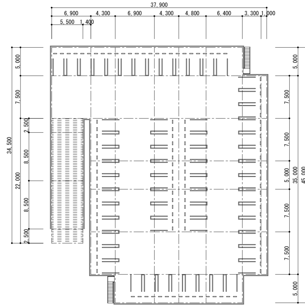
R階平面図
