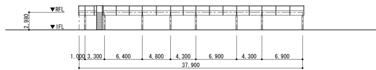
北側立面図
